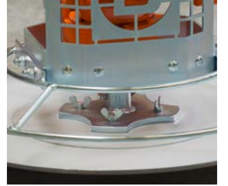
4 kelebek somunların yardımıyla hızlı ve esnek perdah diskleri değiştirebilirsiniz.
